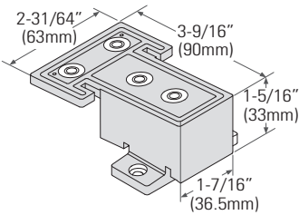
DS725BSPTTBAR tan DS725BSPWTBAR white DS725BSPBLTBAR black For standard T-bar
